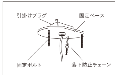
シーリングカップ内側詳細図
